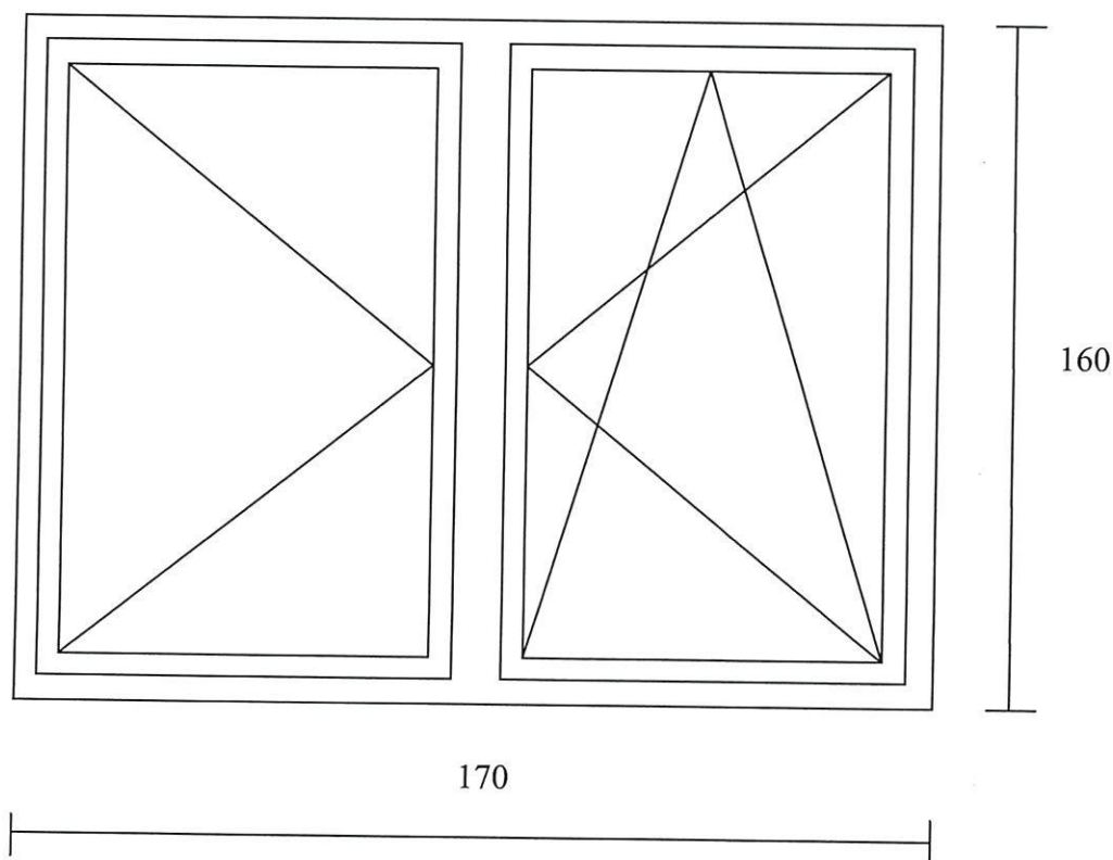
Rys. 1 Stolarka okienna 170x160cm szt. 1
